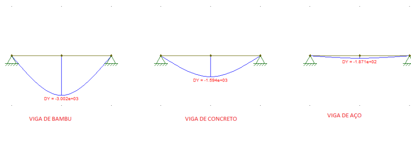
Figura 8 – Resultado dos cálculos realizados pelo Ftool com os elementos na horizontal (Fonte: Próprio autor).
